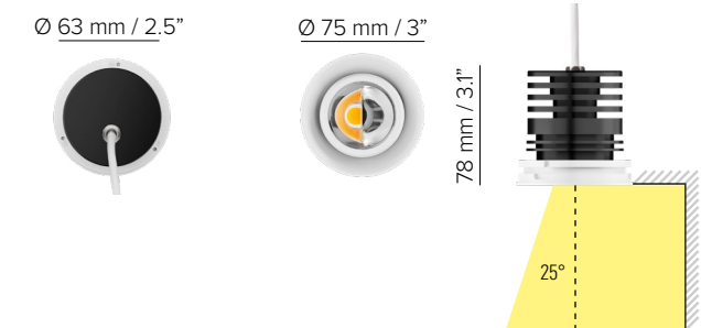
WALLWASHER
